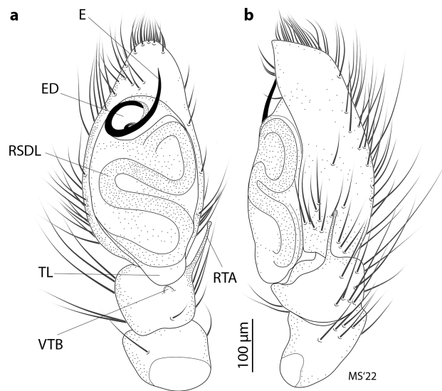
Abb. 14: Euophrys rufibarbis , Männchen aus Frankreich, linker Pedipalpus. a. ventral; b. retrolateral Fig. 14: Euophrys rufibarbis , male from France, left palp. a. ventral view; b. retrolateral view
